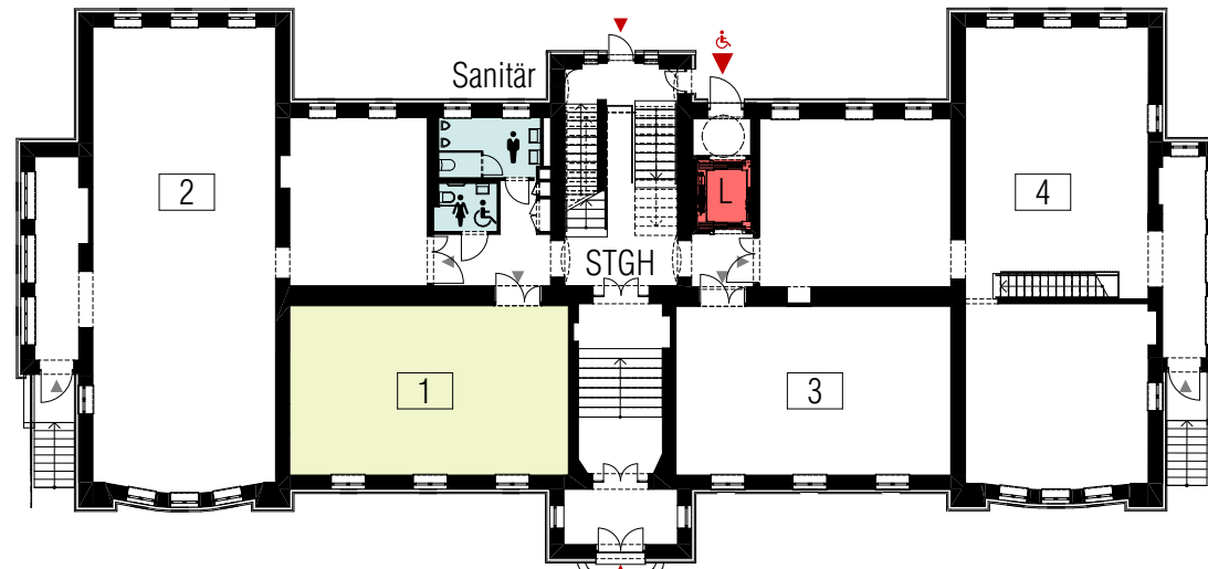
GRUNDRISS ERDGESCHOSS
