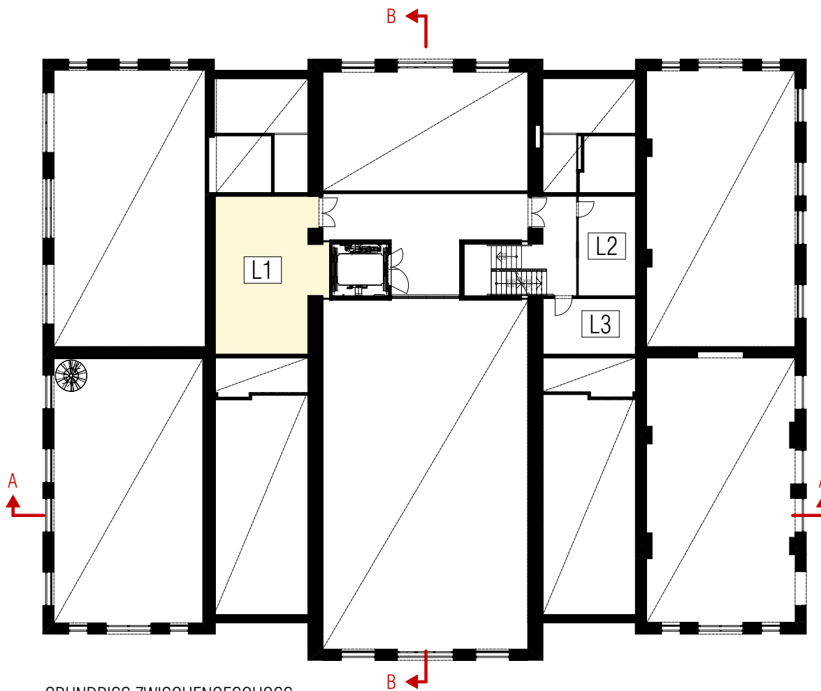
GRUNDRISS ZWISCHENGESCHOSS
