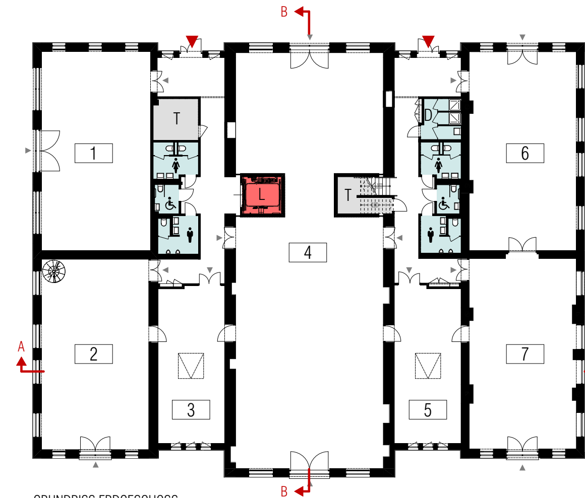
GRUNDRISS ERDGESCHOSS
