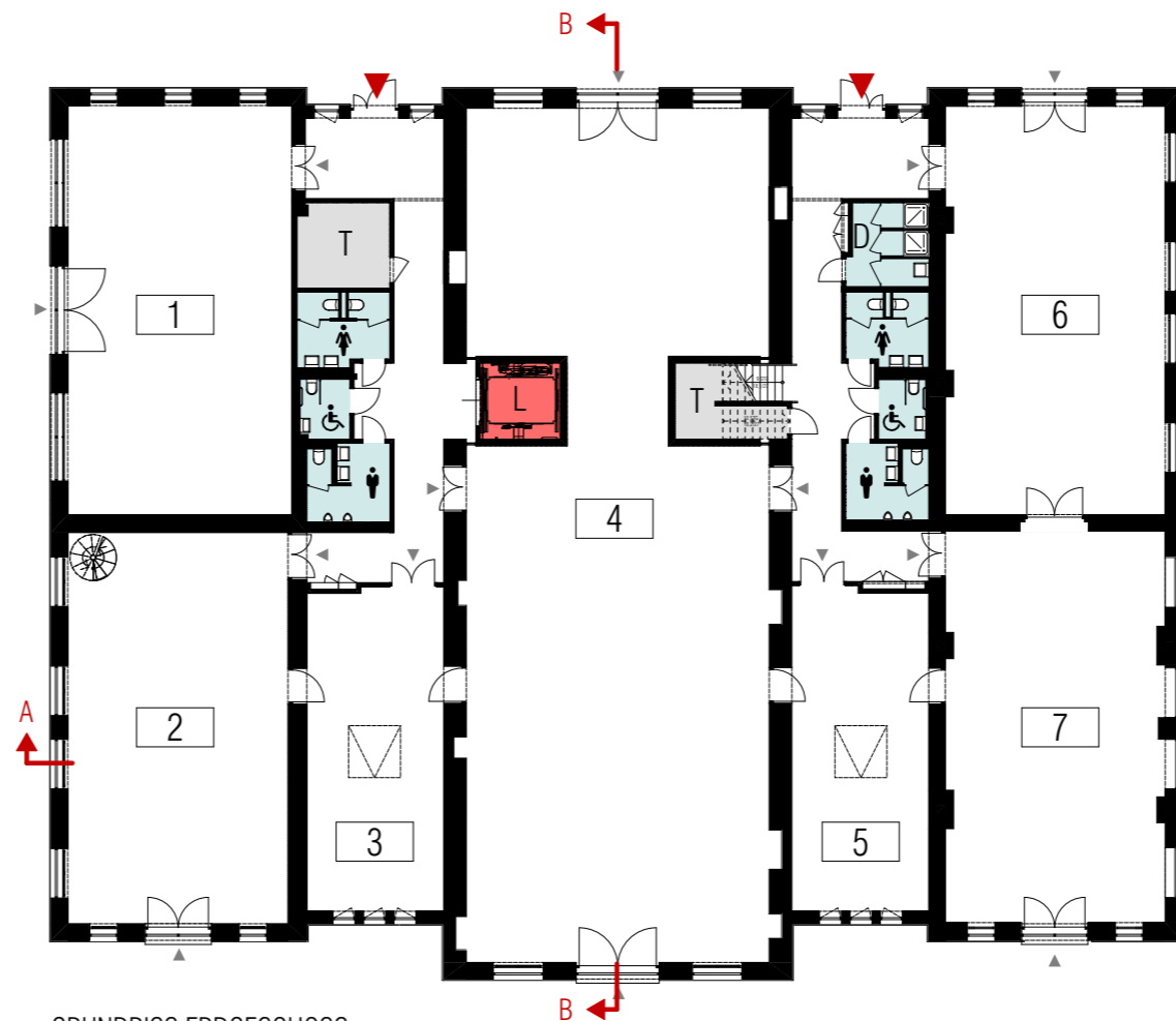
GRUNDRISS ERDGESCHOSS
