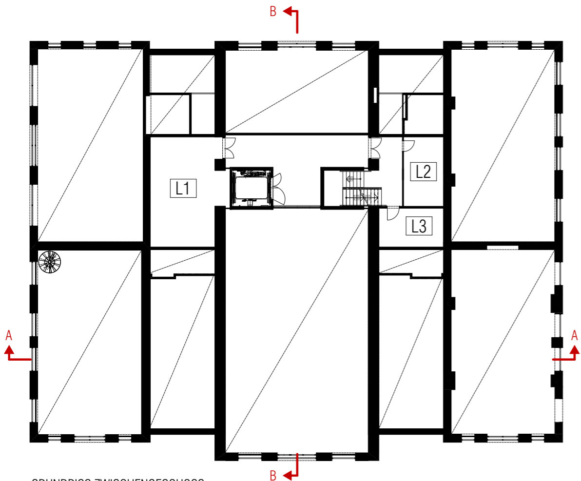
GRUNDRISS ZWISCHENGESCHOSS
