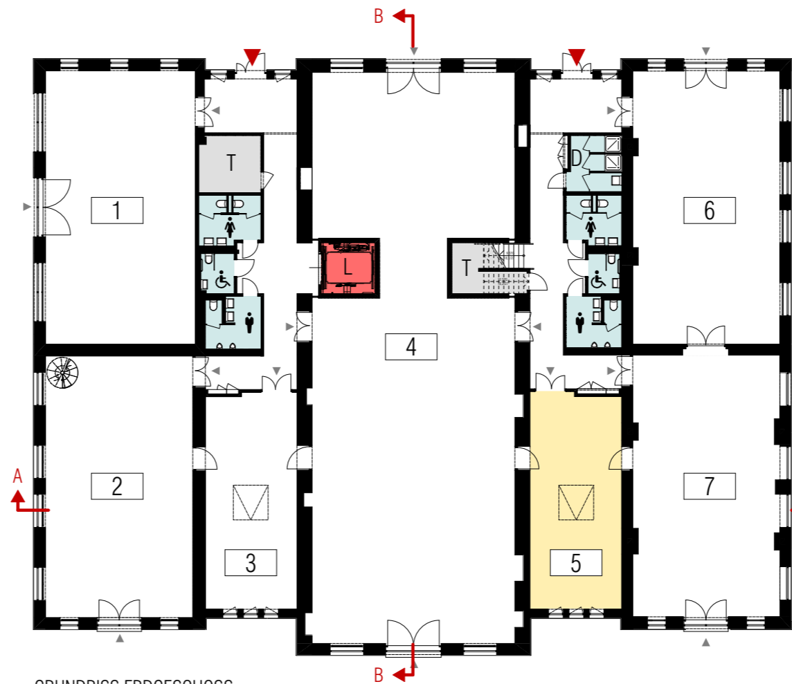
GRUNDRISS ERDGESCHOSS
