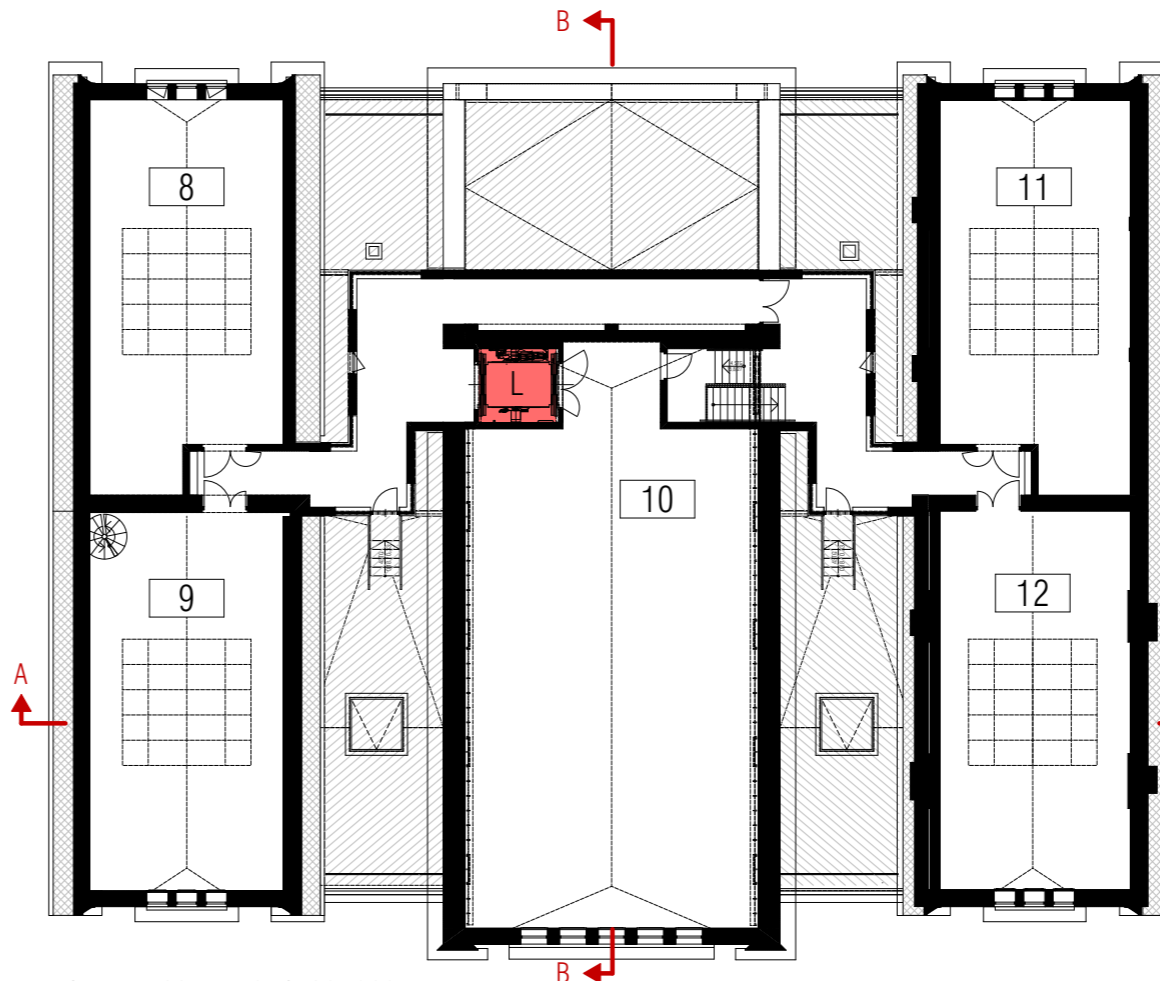
GRUNDRISS 1. DACHGESCHOSS
