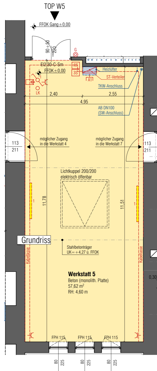
GRUNDRISSAUSSCHNITT ERDGESCHOSS - 1:75 TOP W5
