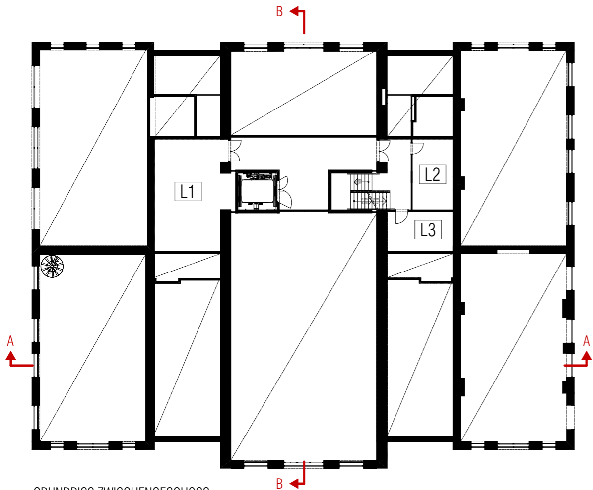
GRUNDRISS ZWISCHENGESCHOSS
