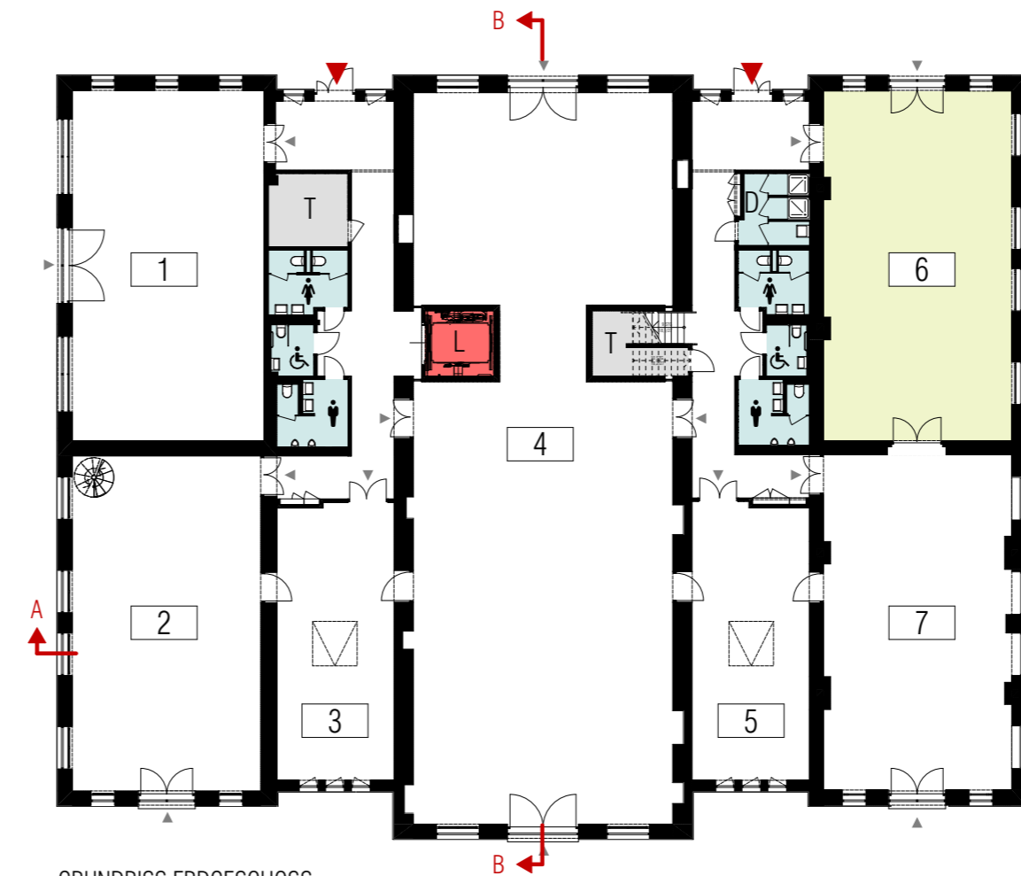
GRUNDRISS ERDGESCHOSS
