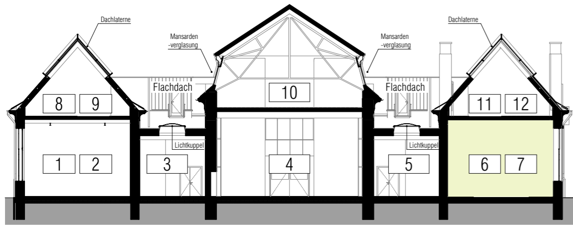
SCHNITT A
