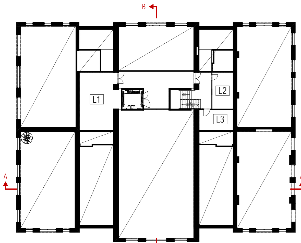
GRUNDRISS ZWISCHENGESCHOSS
