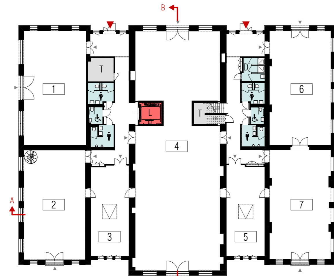
GRUNDRISS ERDGESCHOSS
